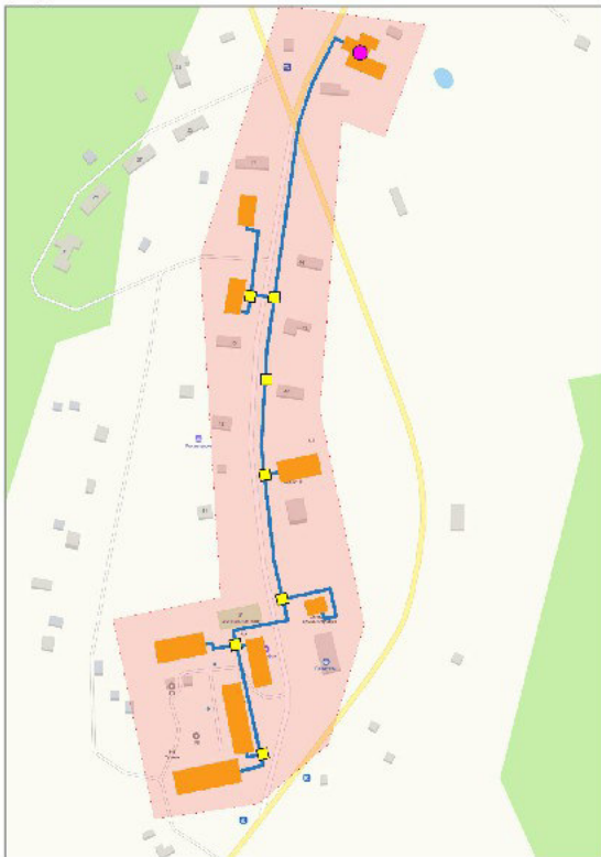
Рисунок 1.4 – Зона действия централизованного теплоснабжения котельной д. Сухое
